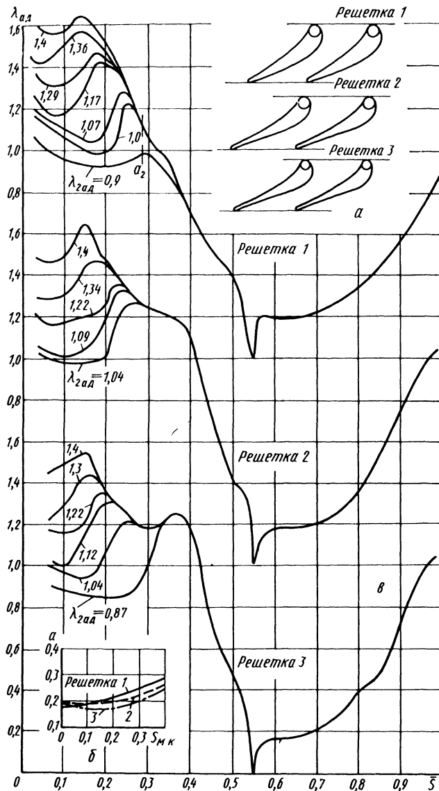
Рис. 5.12. Характеристики решеток 1...3 (табл. 5.1):
