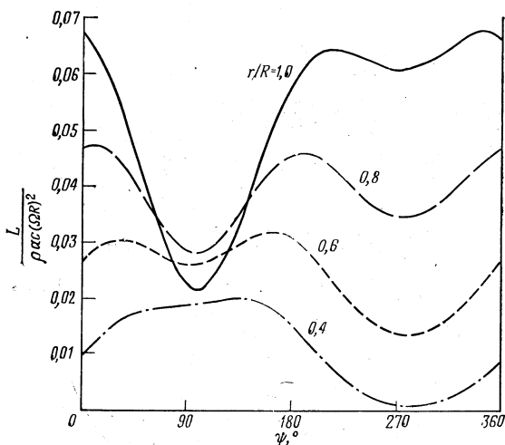
Рис. 5.26. Распределение относительной подъемной силы сечения лопасти по азимуту при \mu = 0,25 , C_T/\sigma = 0,12 , f/A = 0,015 и \theta_{кр} = -8^\circ . Распределение индуктивных скоростей равномерное.
