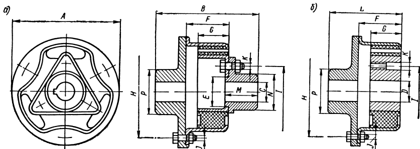
Рис. III.42. Муфта «Кардафлекс»
