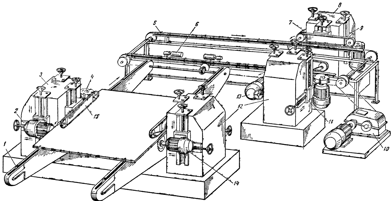
Рис. 121. Схема четырехстороннего форматного станка ЦФ-2:
