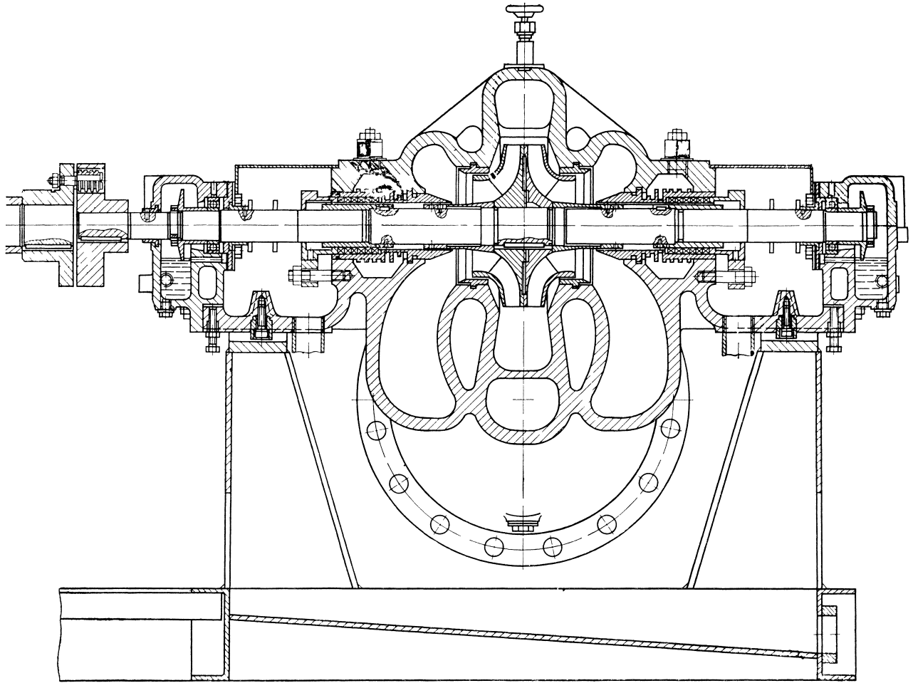
Рис 9-14. Сетевой насос СЭ 500-70.
